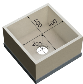
Модель K 400x400
