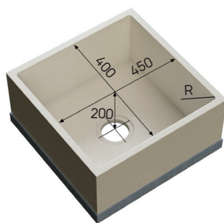
Модель KR 450x400
