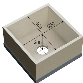
Модель K 500x500
